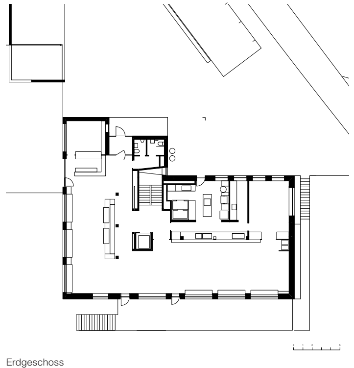
Erdgeschoss
