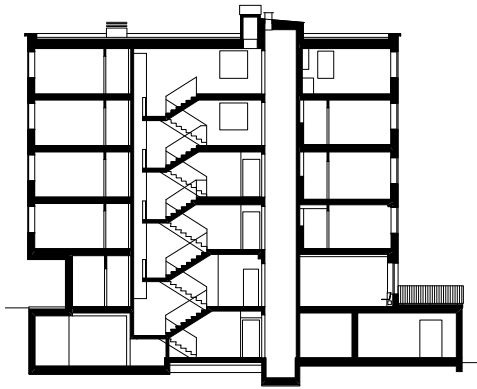
Querschnitt
