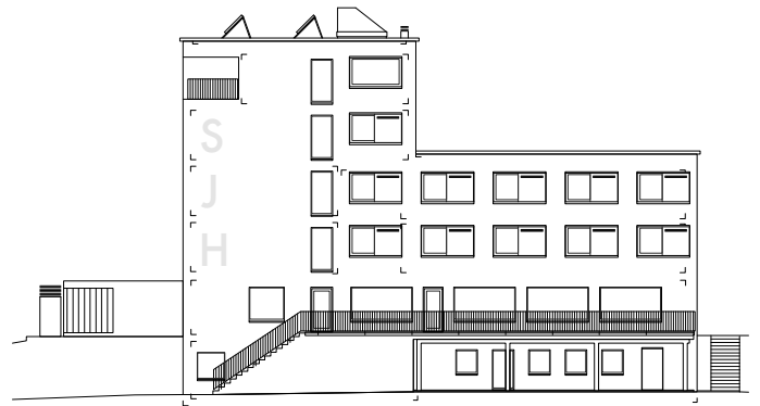
Ostfassade
